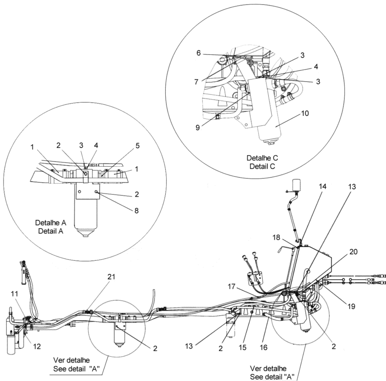
VISTA LATERAL ESQUERDA DO TRATOR LEFT SIDE VIEW THE TRACTOR
